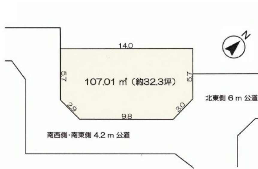
【区画图】
